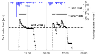
CSO tank dynamics
