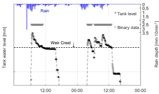
a) CSO tank dynamics
