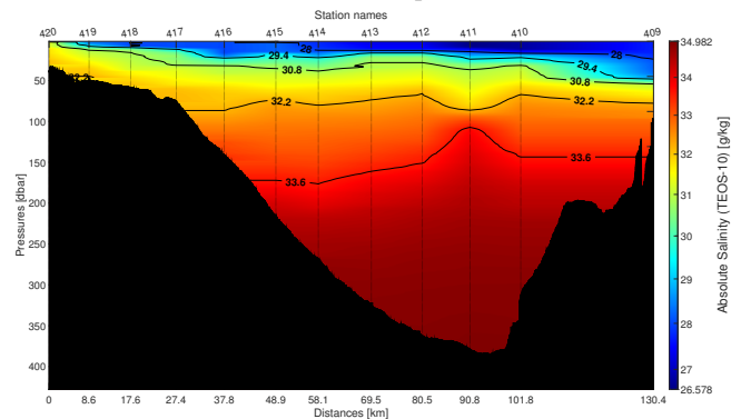
(d) Absolute Salinity [ \text{g/kg} ]
