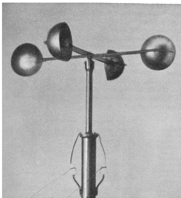
Figure 1. Sandström cup anemometer (Östman, 1928).
