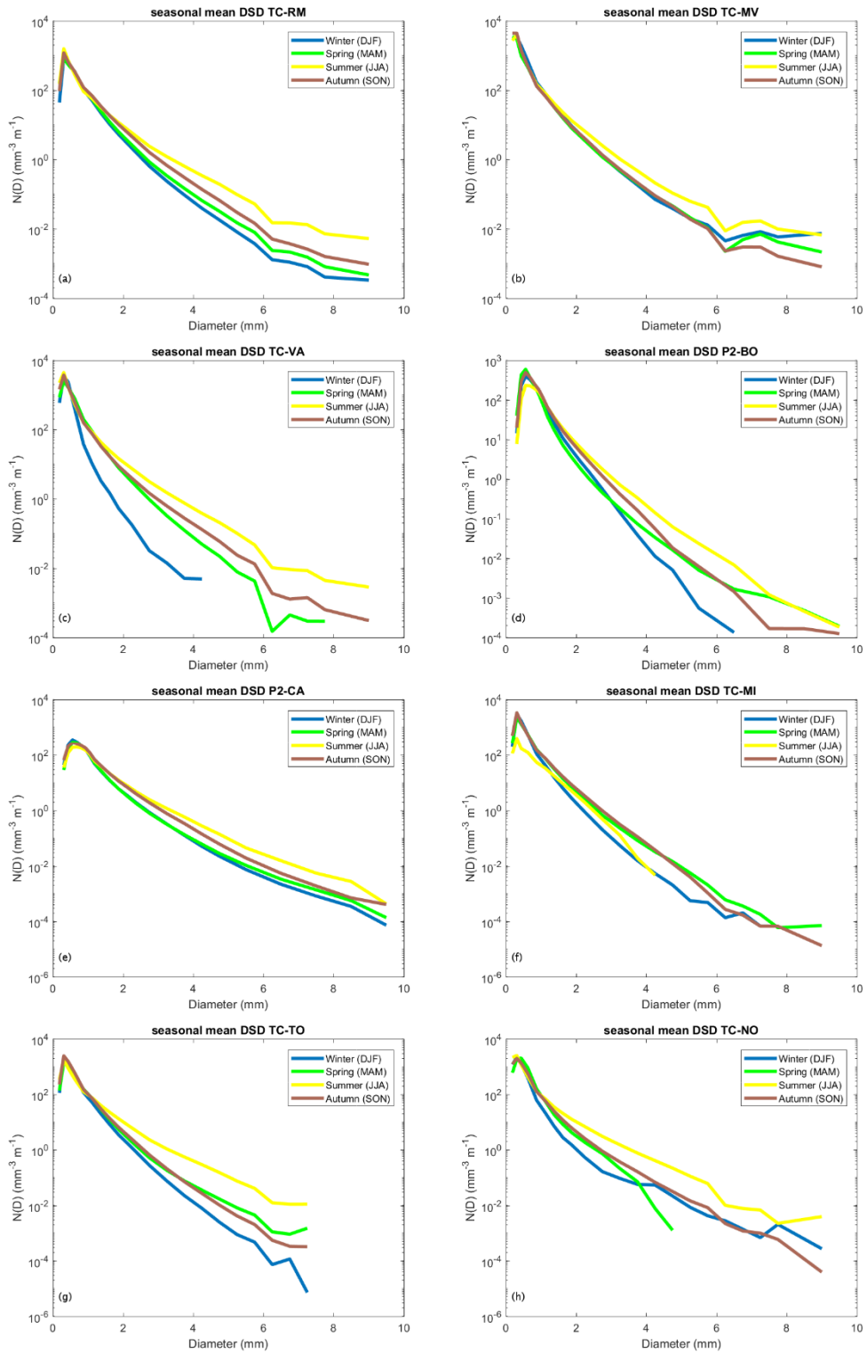
375 Figure 6: seasonal mean DSDs: (a) TC-RM, (b) TC-MV, (c) TC-VA, (d) P2-BO, (e) P2-CA, (f) TC-MI, (g) TC-TO, (h) TC-NO.
