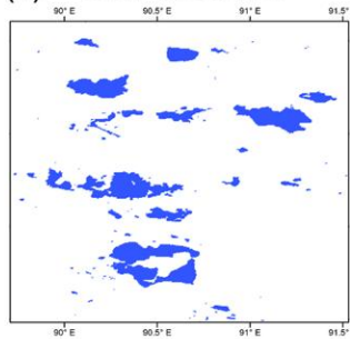
(d) GSWCD DOY200
