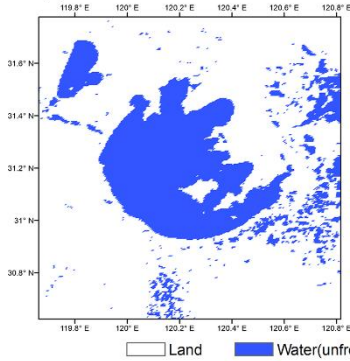
(d) GSWCD DOY001
