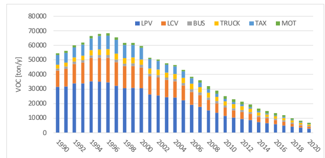
(f) VOC
