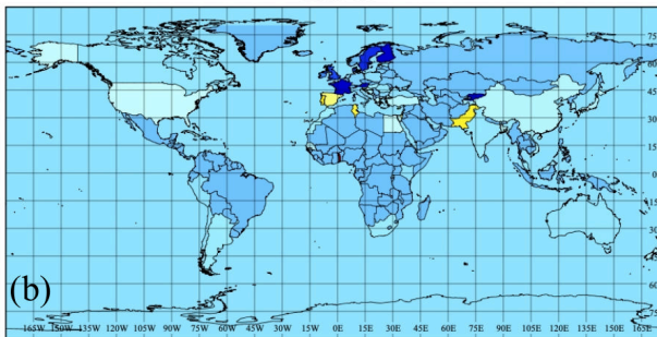
CAMS-GLOB-TEMPO (ene, NMVOC) - August
