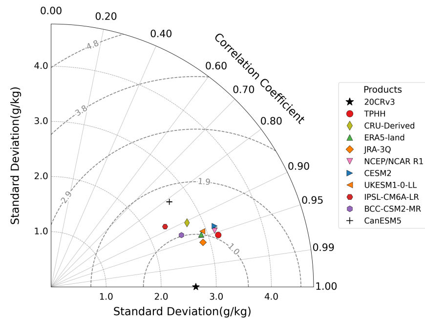
(d) Ref: 20CRv3 (Shum)
