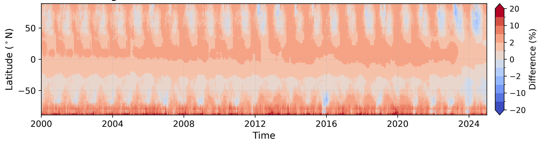
(d) 10 km height
