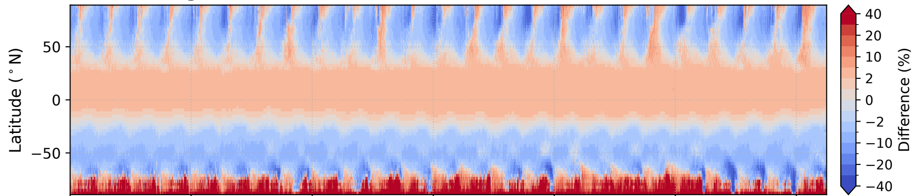
(d) 10 km height
