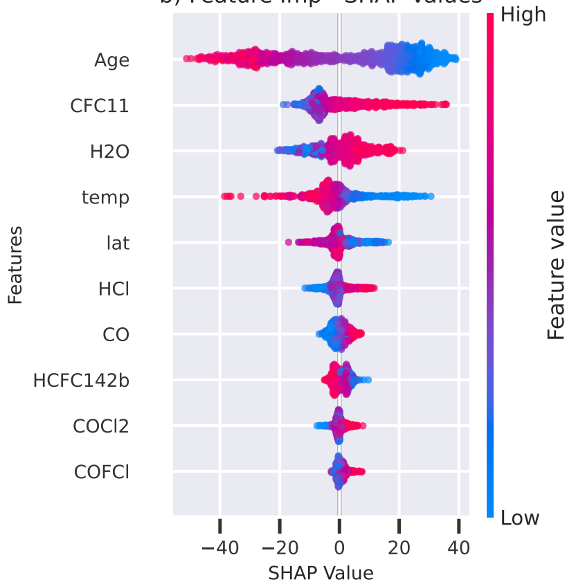
b) Feature Imp - SHAP Values
