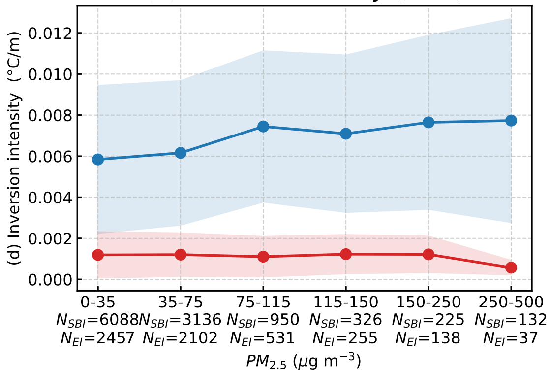
(d) Inversion intensity ( ^{\circ}C/m )
