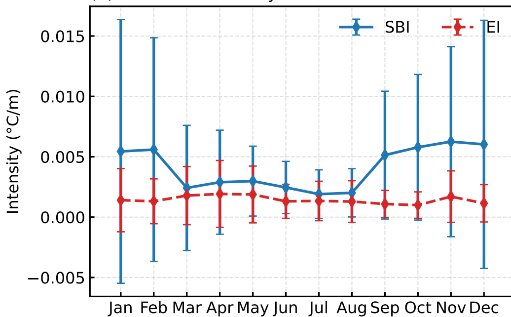
(d) Inversion intensity
