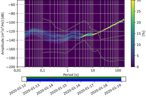
OT.OT05..EHE 2020-01-12 -- 2020-01-18 (333/333 segments)
