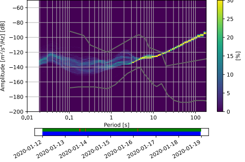
OT.OT05..EHZ 2020-01-12 -- 2020-01-18 (333/333 segments)
