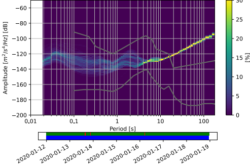
OT.OT05..EHN 2020-01-12 -- 2020-01-18 (333/333 segments)
