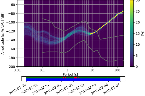
RM.OT07..EHE 2015-01-30 -- 2015-02-06 (383/383 segments)
