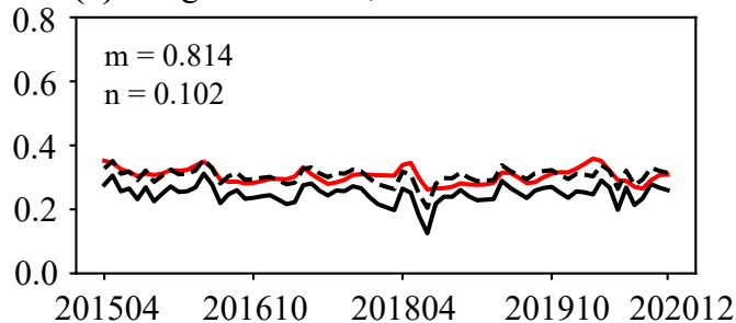
(d) Longitude = 91.7, latitude = 39.2
