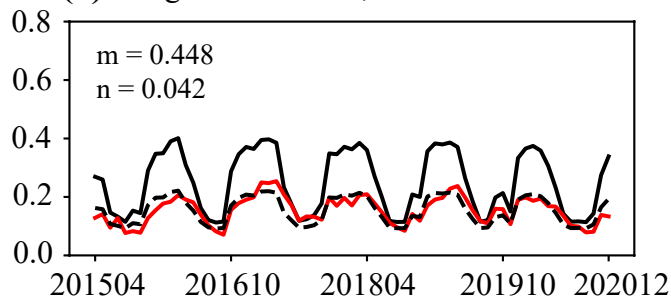
(a) Longitude = -121.0, latitude = 42.1
