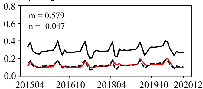
(b) Longitude = 121.3, latitude = 63.8
