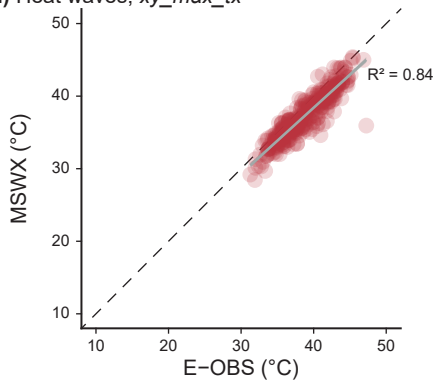
(d) Heat waves, xy_max_tx
