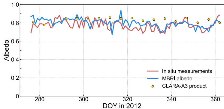
(d) Albedo at Atka AWS2 2012
