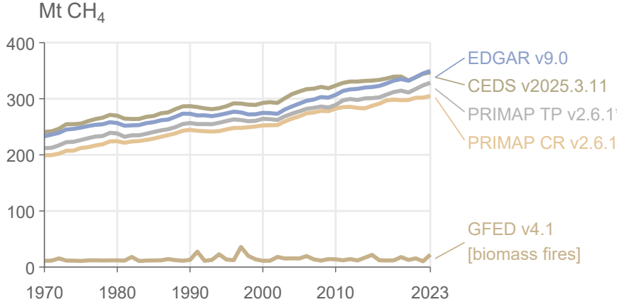
(d) Global CH 4 emissions
