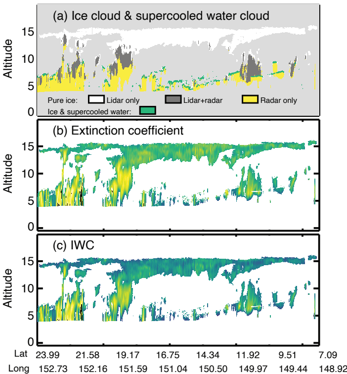
DARDAR (V3.10)
