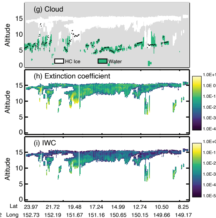
CALIOP (V4.20 CPro)
