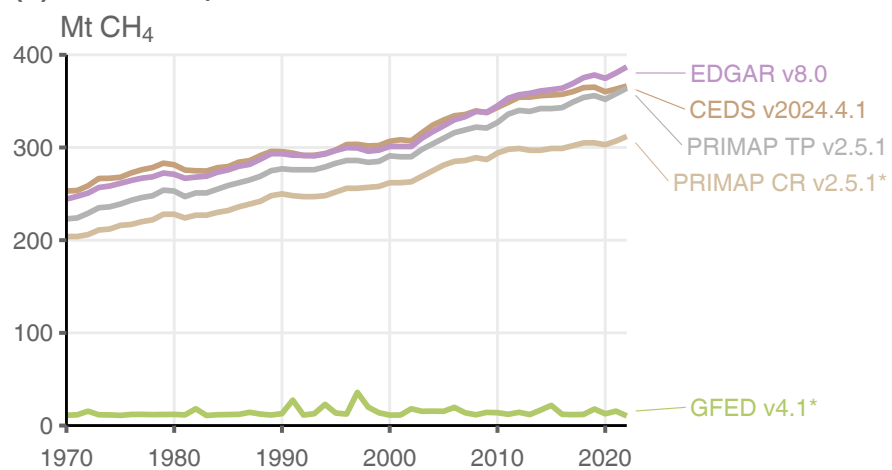
(d) Global CH 4 emissions
