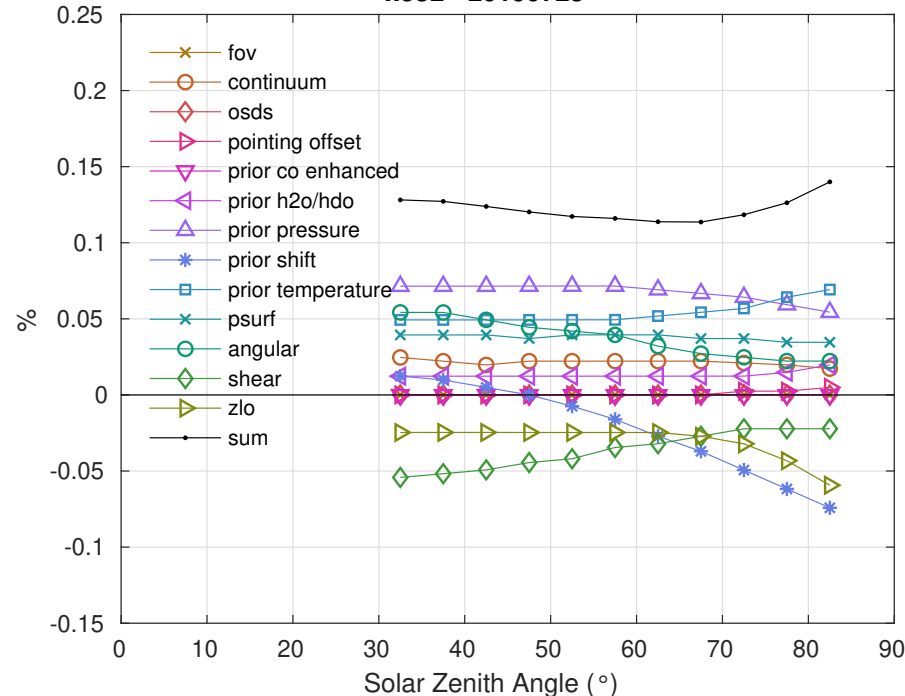
xco2 - 20190723
