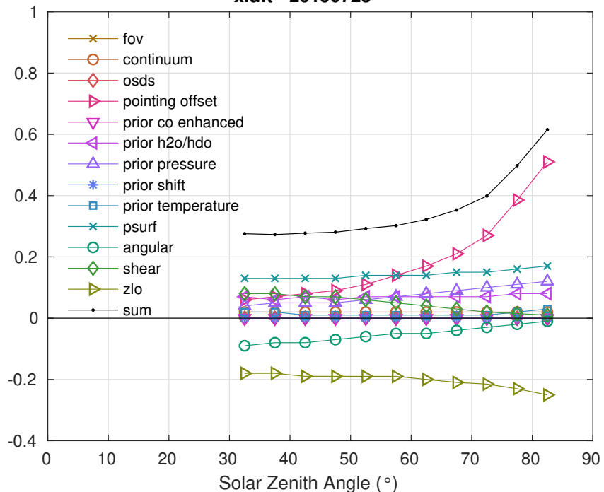
xluft - 20190723
