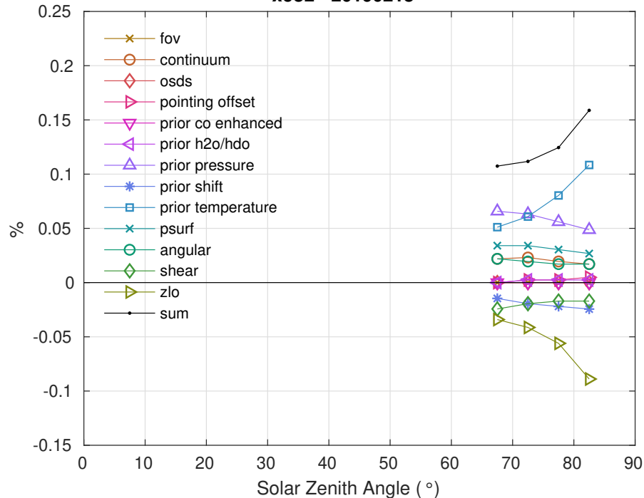
xco2 - 20190218
