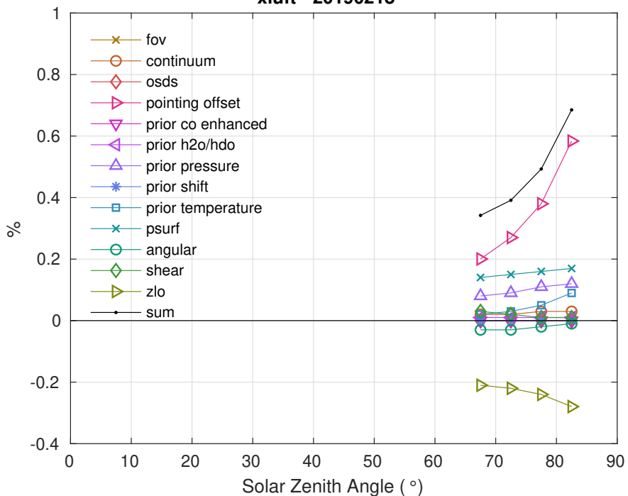
xluft - 20190218
