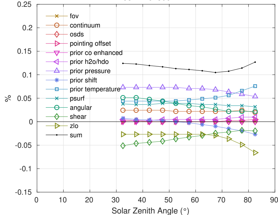
xco2 - 20190611
