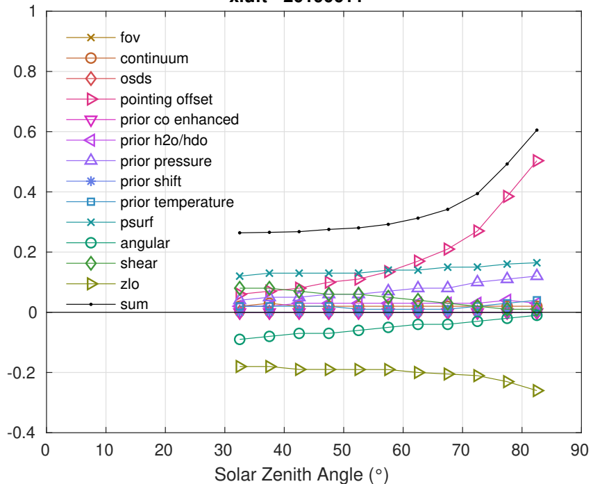
xluft - 20190611
