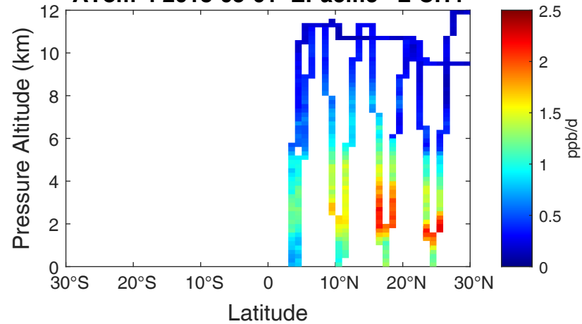
ATom-4 2018-05-01 EPacific L-CH4
