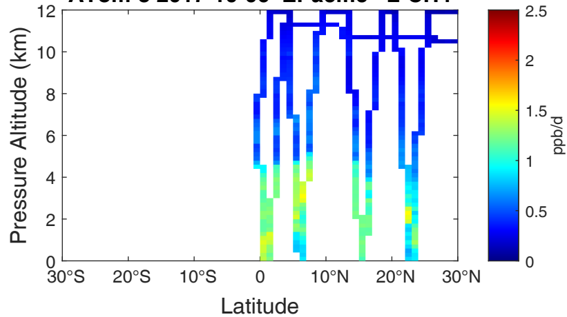
ATom-3 2017-10-06 EPacific L-CH4
