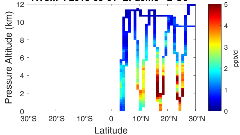
ATom-4 2018-05-01 EPacific L-O3
