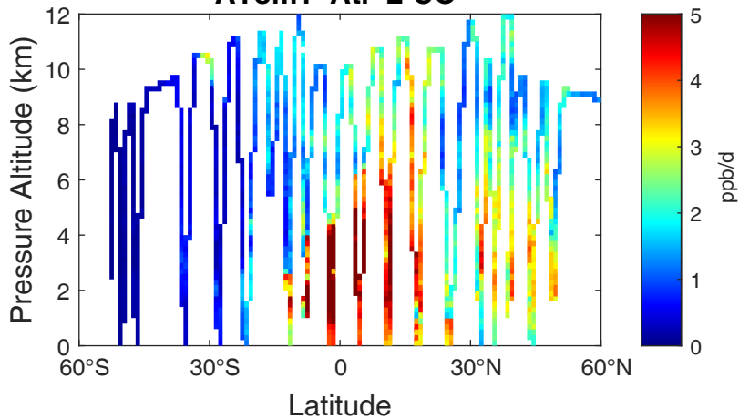
ATom3 Atl L-CO
