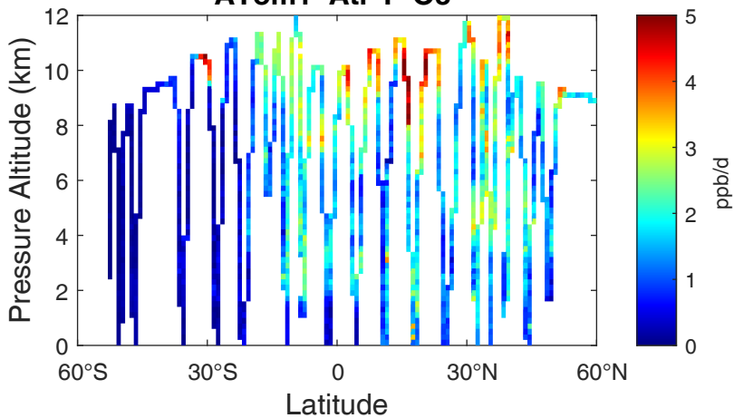
ATom3 Atl P-O3
