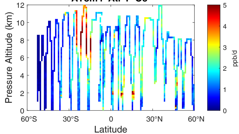
ATom4 Atl P-O3
