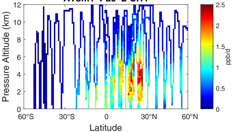
ATom3 Pac L-CH4
