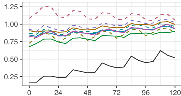
(d) Spread-error-ratio
