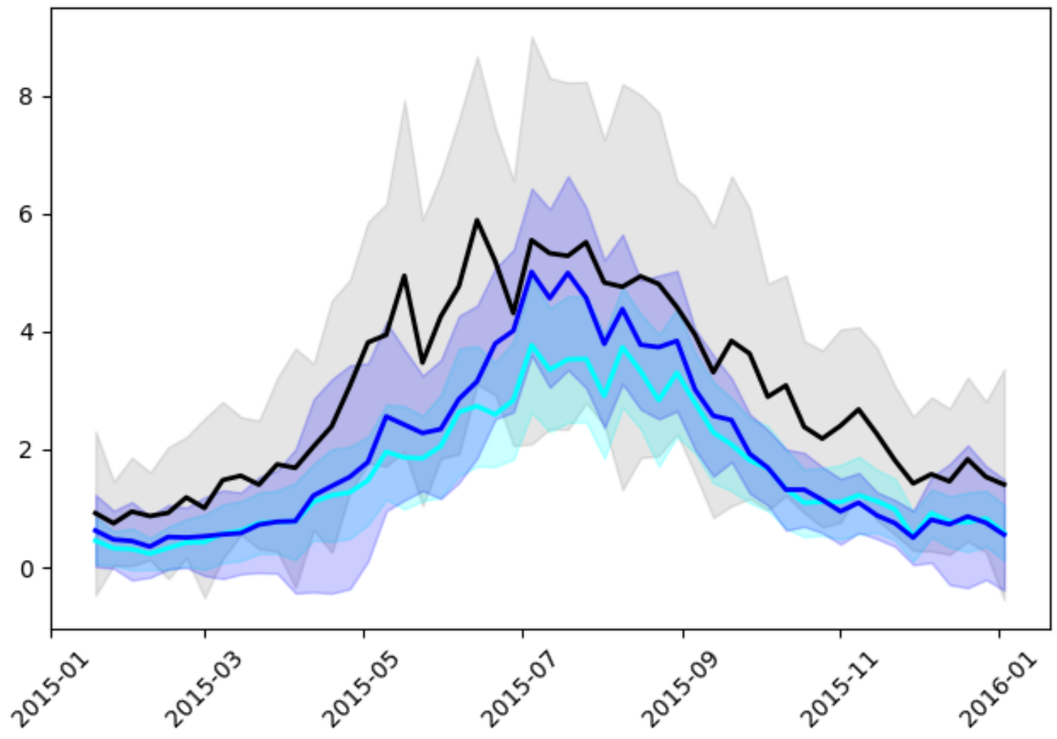
(c) REC ( \mu\text{molm}^{-2}\text{s}^{-1} ) nsites=25
