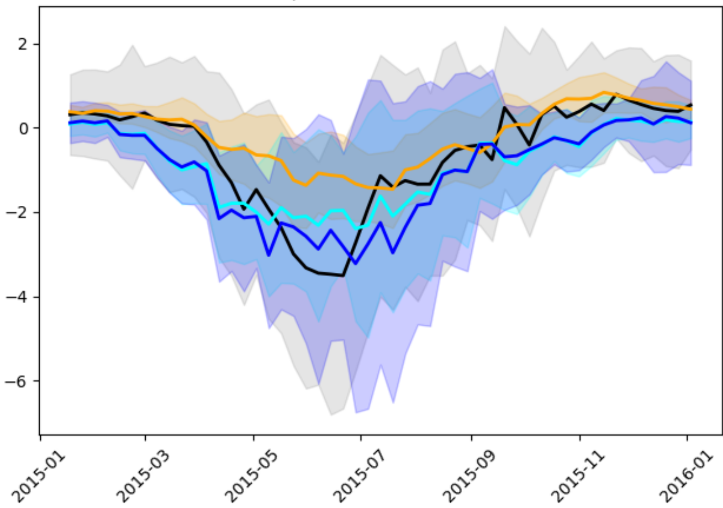
(a) NEE ( \mu\text{molm}^{-2}\text{s}^{-1} ) nsites=25
