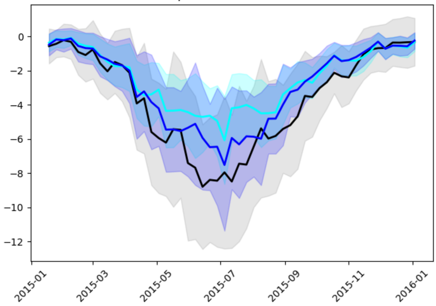
(b) GPP ( \mu\text{molm}^{-2}\text{s}^{-1} ) nsites=25
