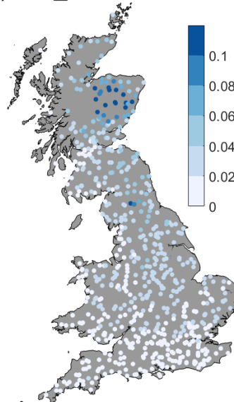
e) frac_snow
