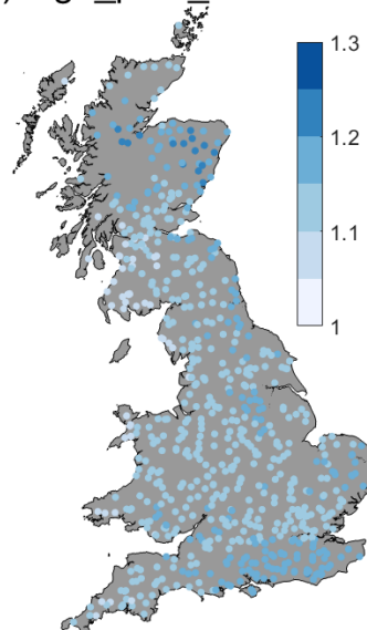
g) high_prec_dur
