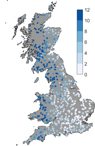
i) Q95
