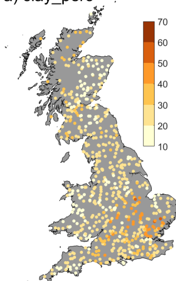
a) clay_perc
