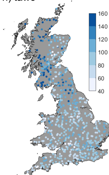
h) tawc
