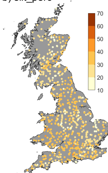
b) silt_perc
