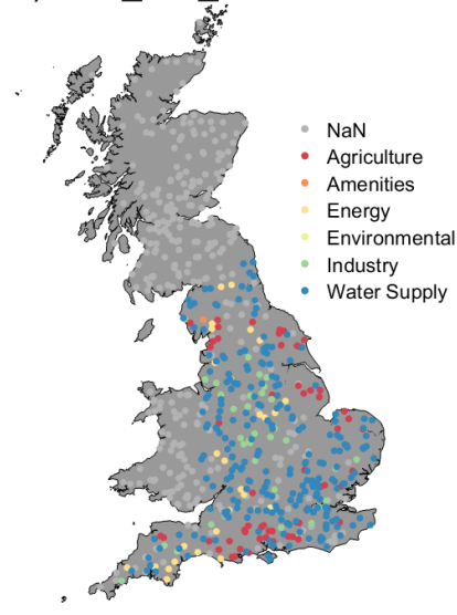
e) dom_abs_use
