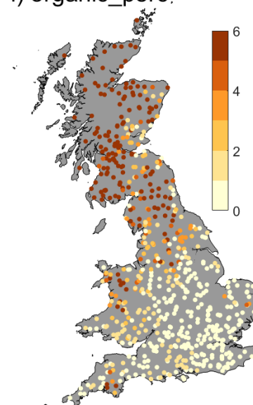
i) organic_perc
