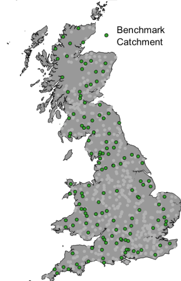
a) benchmark_catch
