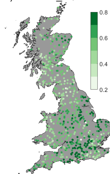
h) Q5
