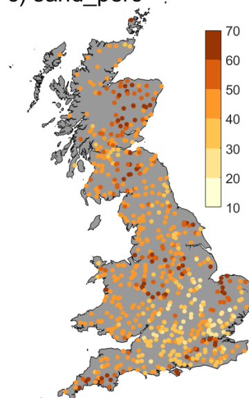
c) sand_perc
