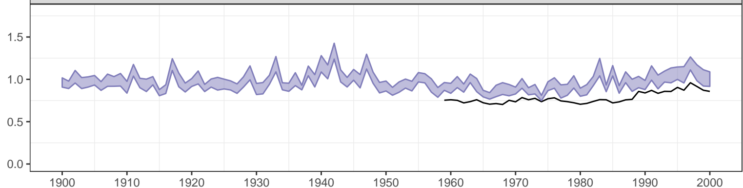
RMSE (° C)
