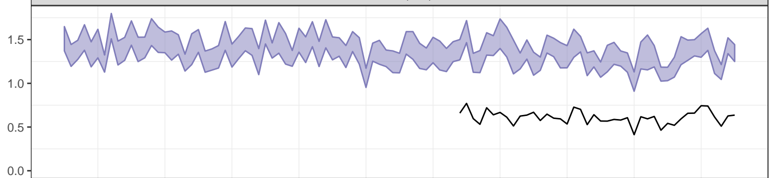
RMSE (° C)
