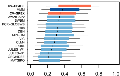
R^2_{anom}
