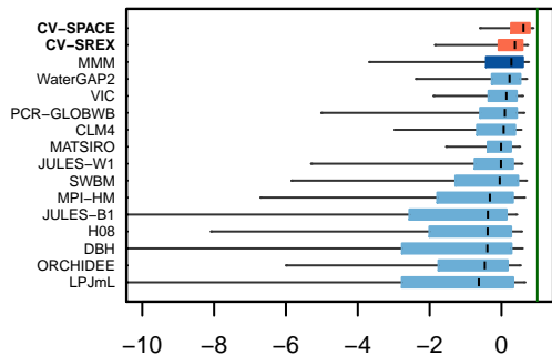
NSE
