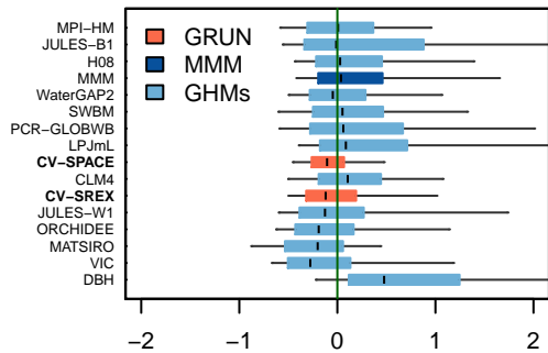
relBIAS
