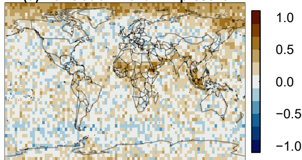
(d) Correlation: 7040 BP–present
