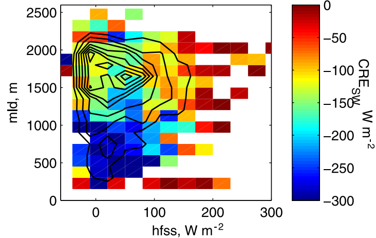
(d) \text{CRE}_{\text{SW}} JJA pm
