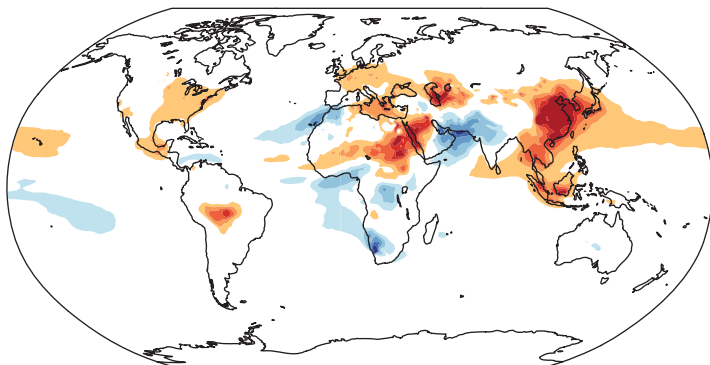
(d) Aerosol forcing (surface)
